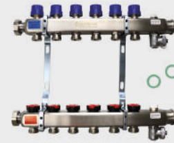
Verteiler Edelstahl 1" Typ Durchflussmengenbegrenzer
